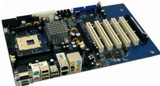
986LCD-M/ATXE
